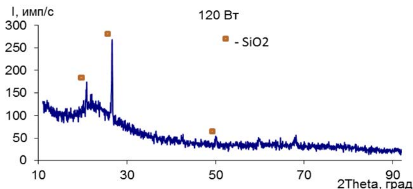
Рис. 2. Дифрактограмма образца, полученного после воздействия лазерного излучения мощностью 120 Вт.
