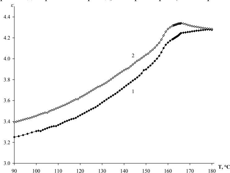
Рис. 2. Температурная зависимость диэлектрической проницаемости образца NaNO_2/Al_2O_3 (100 нм) на частоте 3 МГц: 1 – нагрев; 2 – охлаждение
