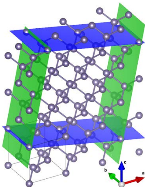
Рис. 1. Примитивная ячейка (ограничена синими и зелеными плоскостями сечения) с гранью (105) (синяя плоскость) в кристаллическом германии.
