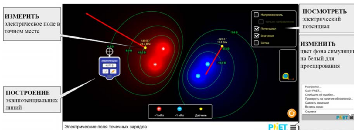
Рис. 2. Лабораторная работа «Электрические поля точечных зарядов», визуализация потенциала для случая +2 нКл и -2 нКл
