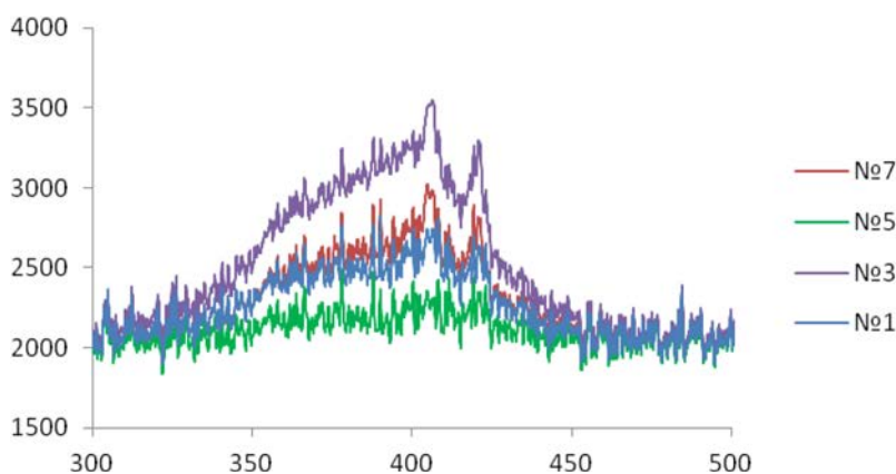
Рис. 3. Спектры люминесценции углеродных соединений: № 1 – Soot; № 3 – C 60 ; № 5 – нанотрубки; № 7 – C 60/70 .
